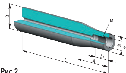
Рис.2 Цилиндрический хвостовик.
