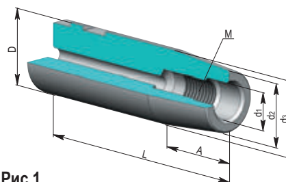
Рис.1 Хвостовик «Weldon».
