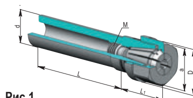
Рис.1 Хвостовик с упором. Шестигранная гайка.
