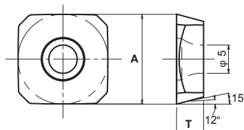
Рис. 2 (чистовая обработка)
