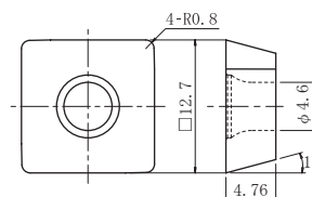
SDHW1204PDTR Без стружколома Сплав: JC8015
