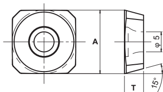
Рис. 1 (чистовая обработка)
