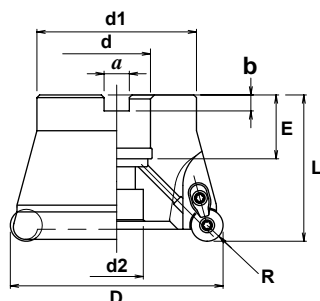
Рис. 1 - Стандартный шаг
