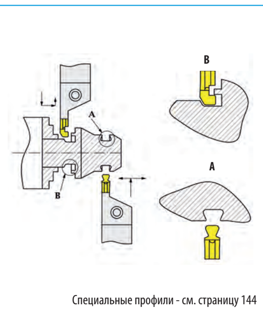
Пример обработки высокоточных канавок
