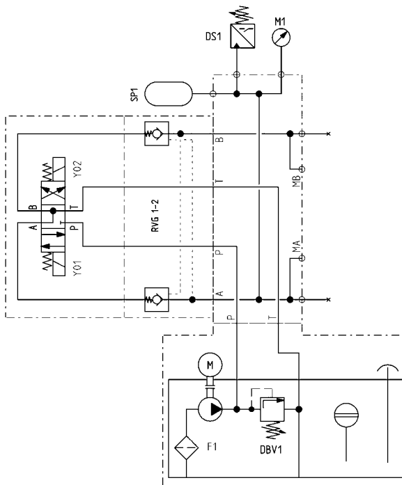
ZRP 2,5 : Q = 2,5 l/min., n = 1450 U/min. Tank volume: V=10 l
